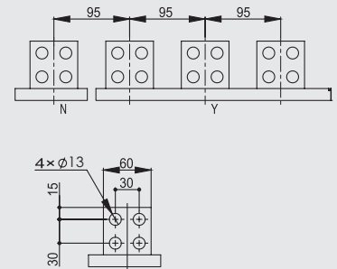
详图
