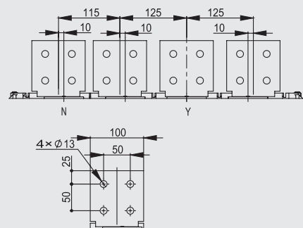
固定详图
