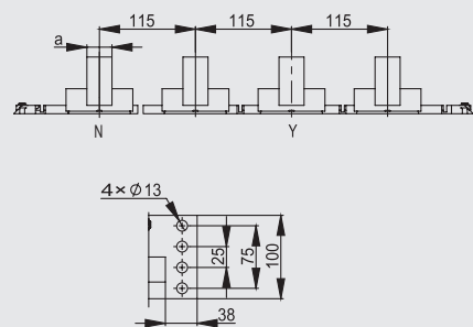
详图
