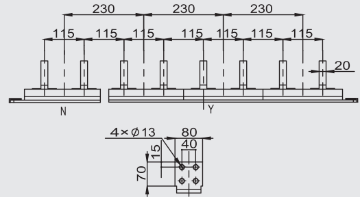
详图
