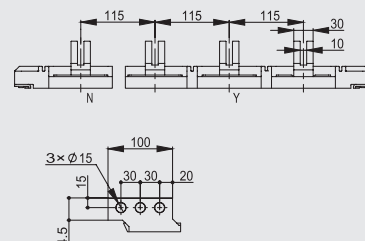
详图
