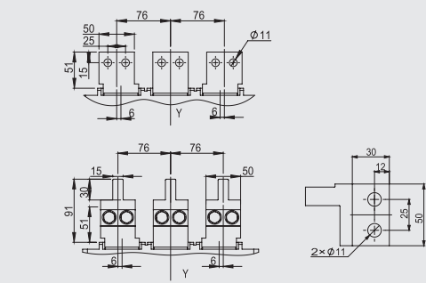
详图
