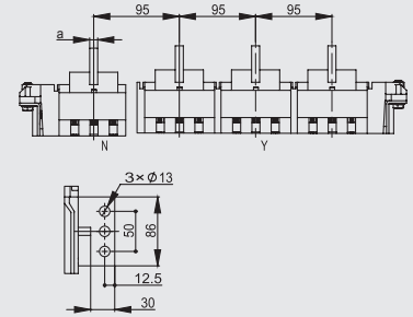
详图
