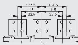
详图
