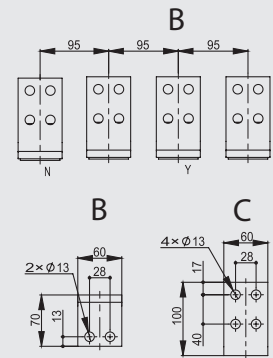
详图
