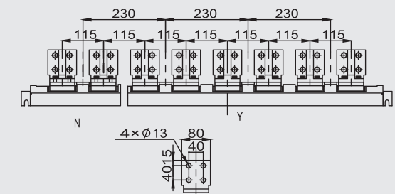
详图
