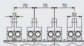
固定详图
