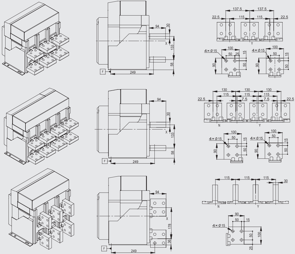
详图
