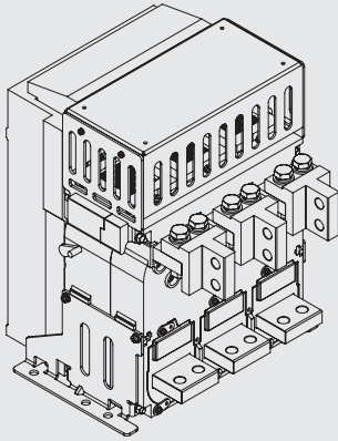
上垂直下水平接线
