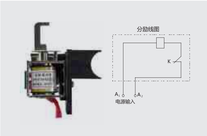
分励脱扣器接线图
