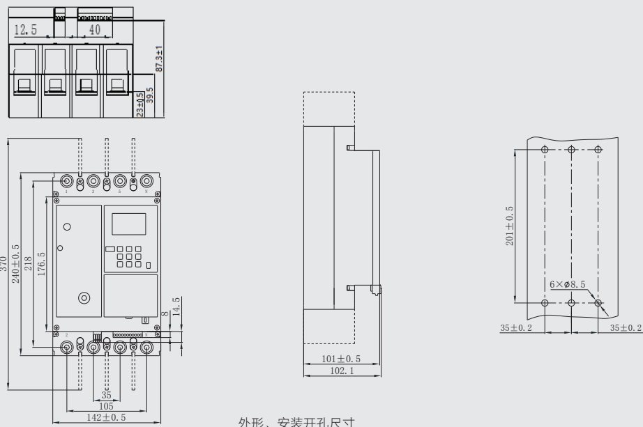
外形、安装开孔尺寸
