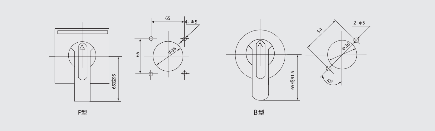
125/250/400/630手柄安装孔示意图
