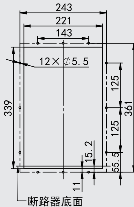
抽屉式
