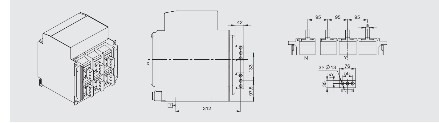
垂直接线
