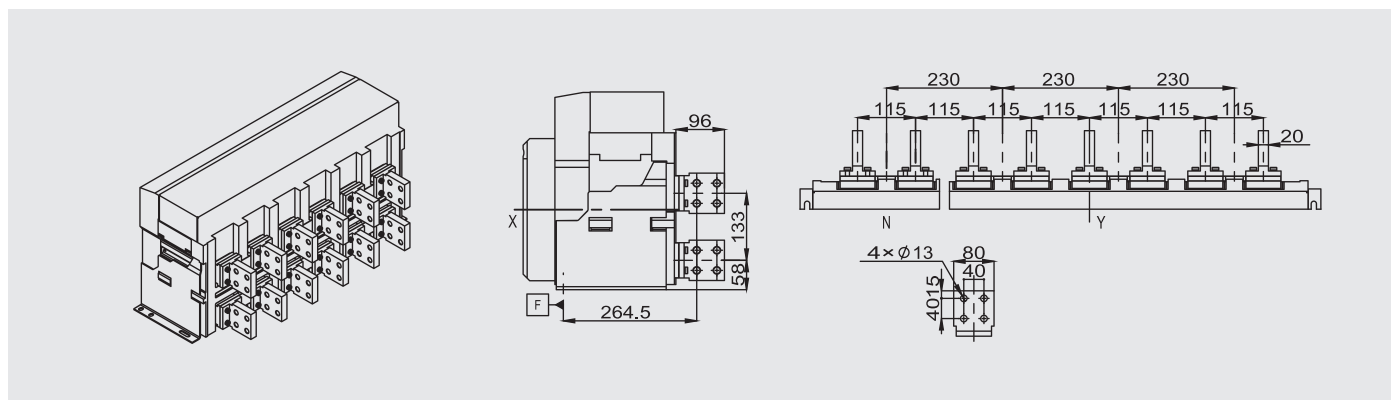
垂直加长接线
