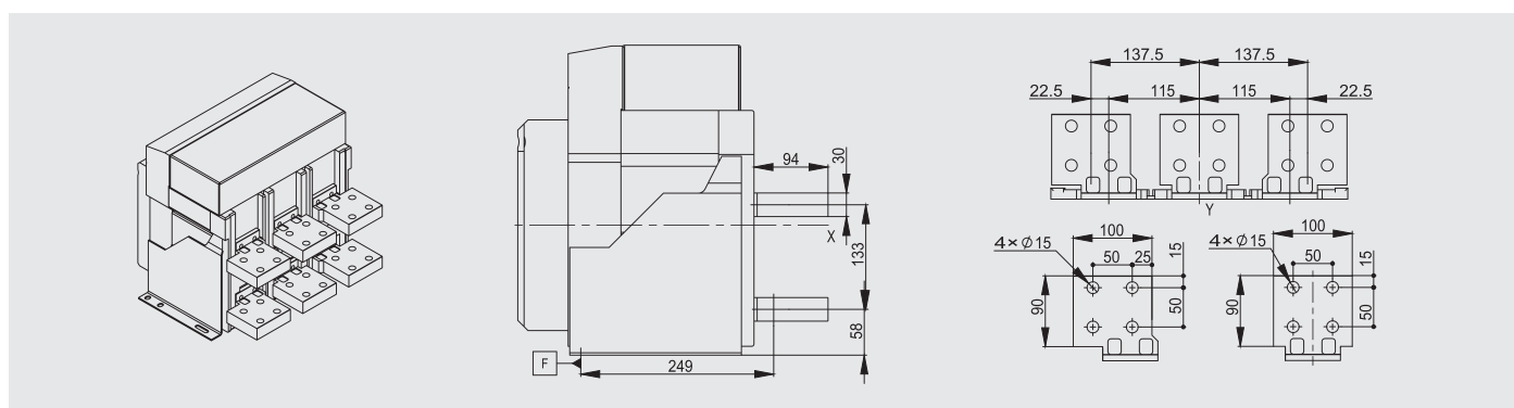
3200A-4000A水平加长、垂直加长接线
