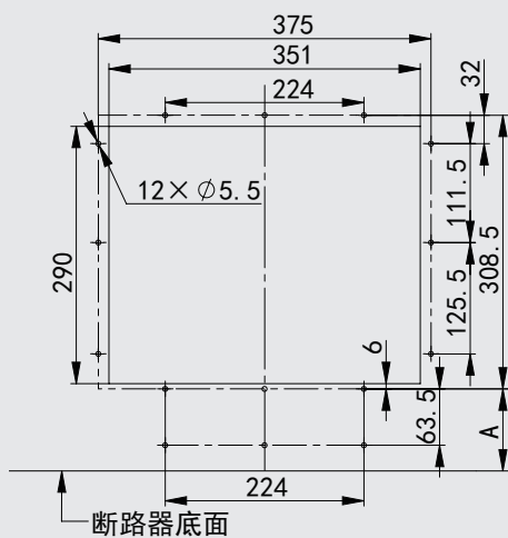
固定式
