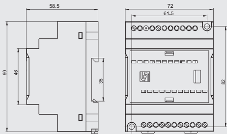
继电器模块安装图
