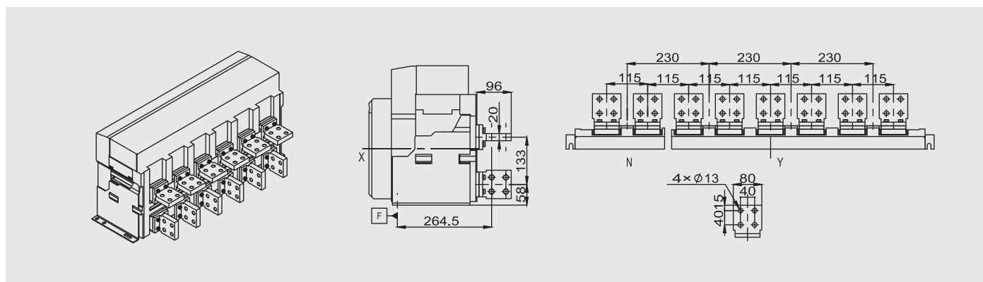
混合加长接线（上水平下垂）
