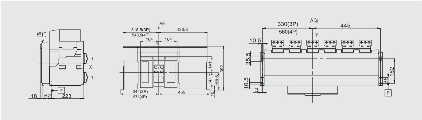
尺寸
