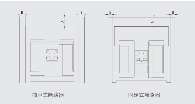
单位：mm
