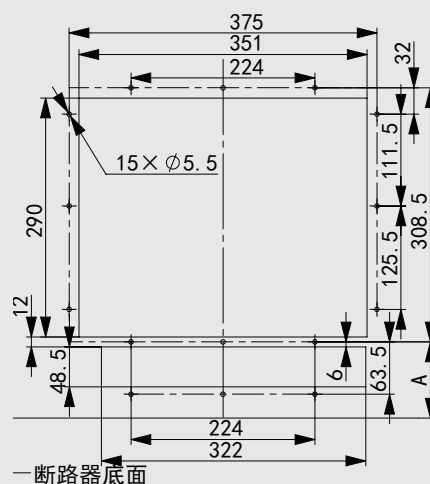
抽屉式
