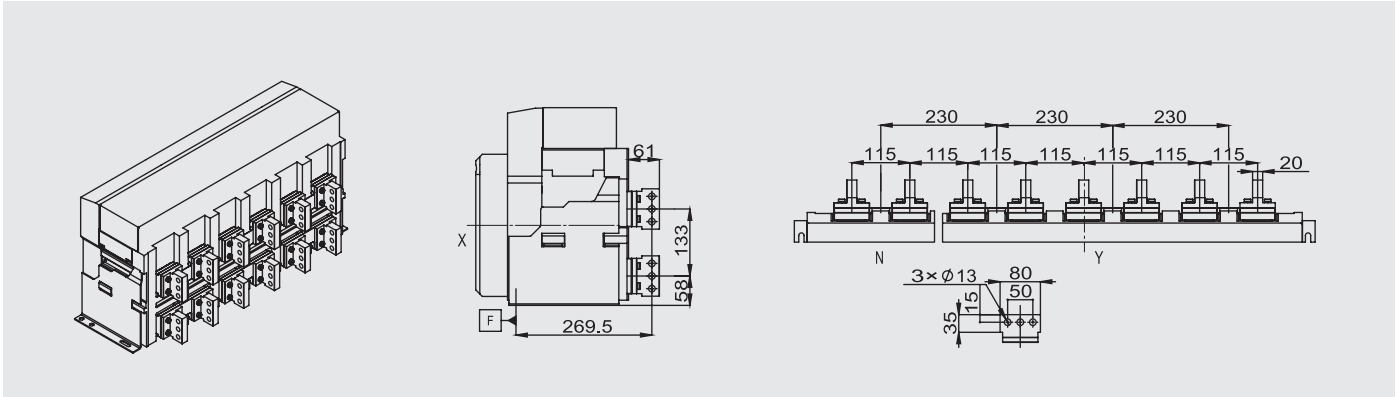
垂直接线
