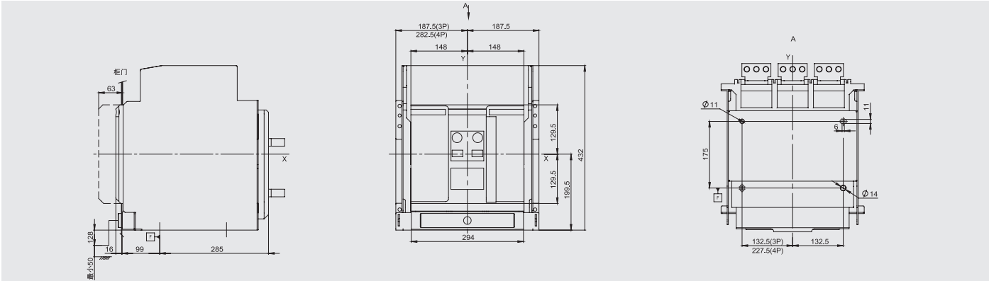
详图
