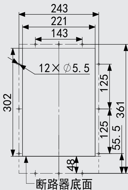
固定式
