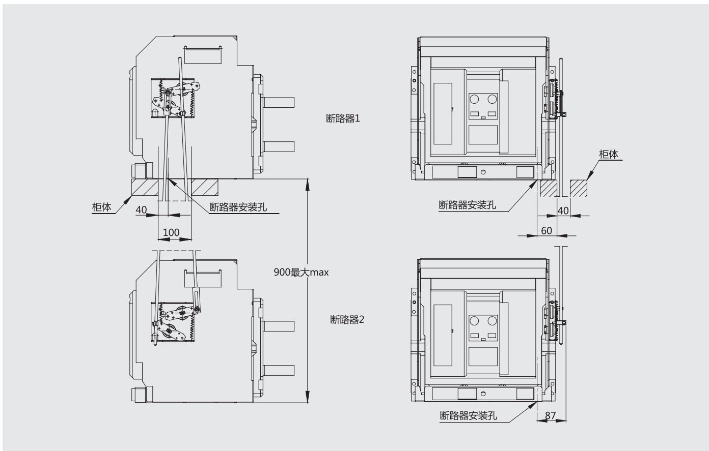
安装示意图：（一合一分）
